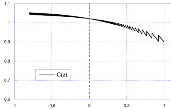
(d) Nominal debt: C(z) for \sigma = 1.0
